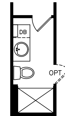
OPTIONAL SHOWER
